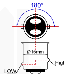
BAY15D-(P21/5W)
