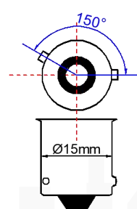
BAU15S-(PY21W)
