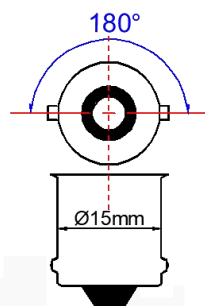
BA15S-(P21W)
